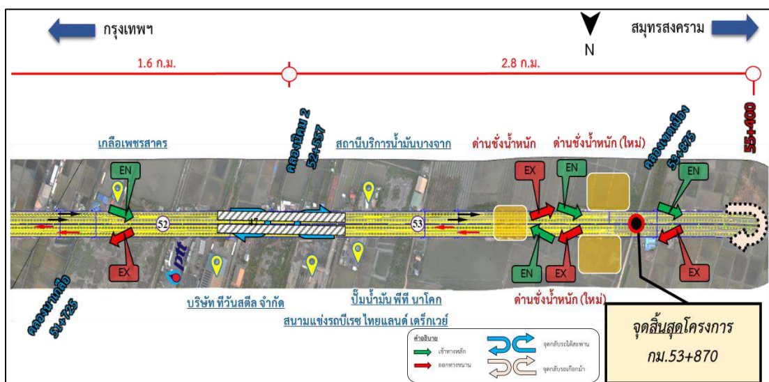
รูปที่ 5-13 ตำแหน่งจุดเข้า-ออกทางหลักและทางขนาน (ต่อ)
