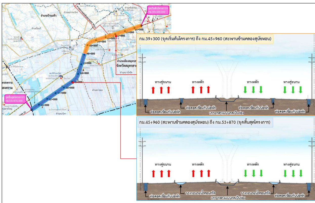
รูปที่ 5-16 ตัวอย่างงานออกแบบระบบระบายน้ำบริเวณพื้นที่โครงการ
