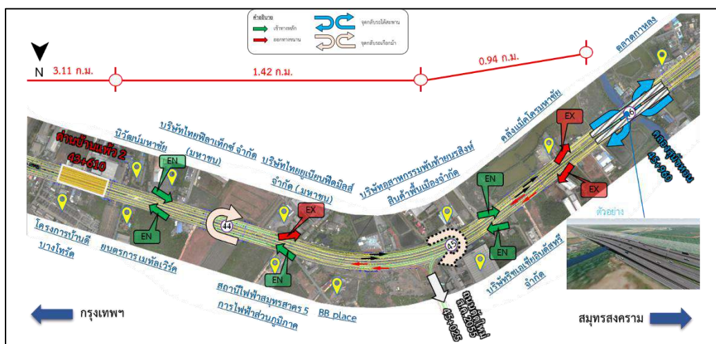
รูปที่ 5-13 ตำแหน่งจุดเข้า-ออกทางหลักและทางขนาน
