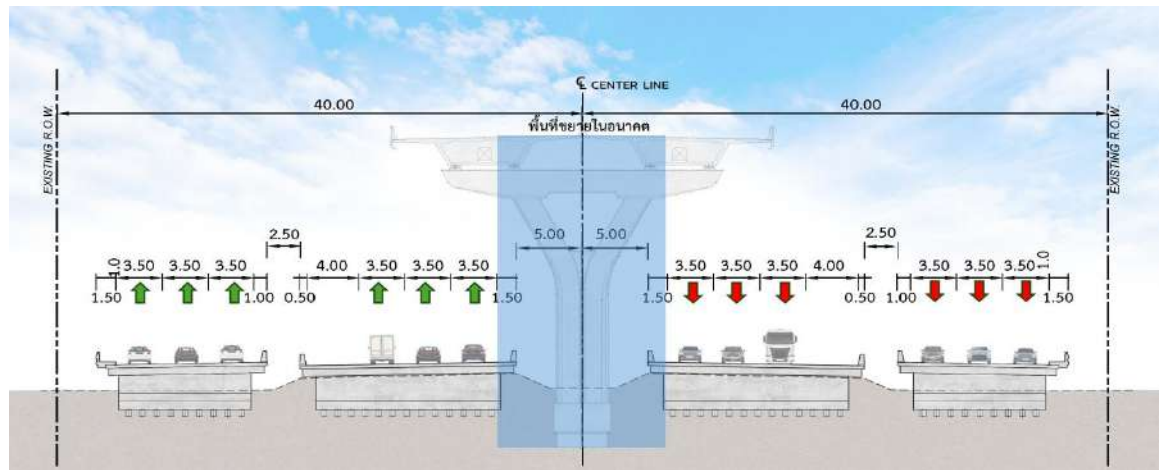
รูปที่ 5-3 ตัวอย่างรูปแบบทั่วไปของถนนโครงการช่วงบริเวณสะพานข้ามคลอง
