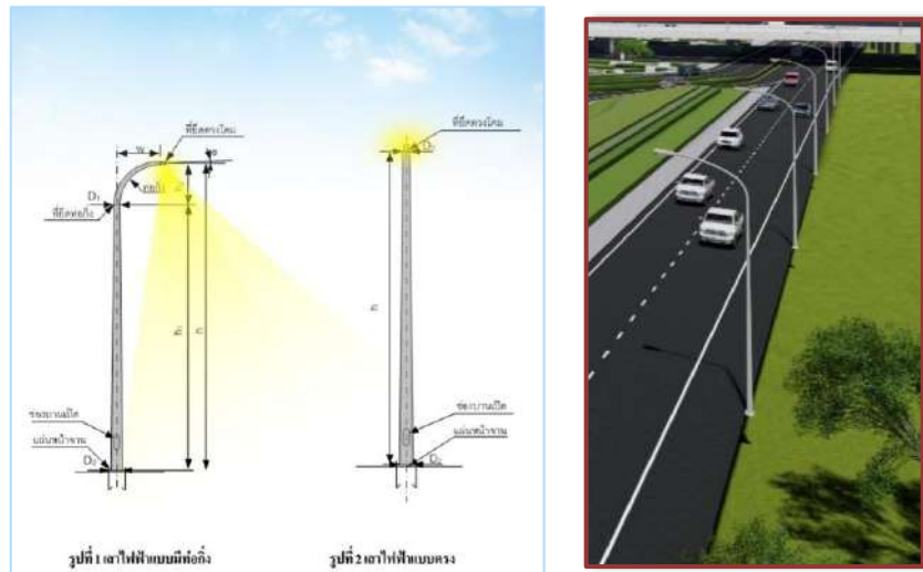
รูปที่ 5-17 ตัวอย่างเสาไฟฟ้าแสงสว่างแบบกิ่งเดี่ยว
