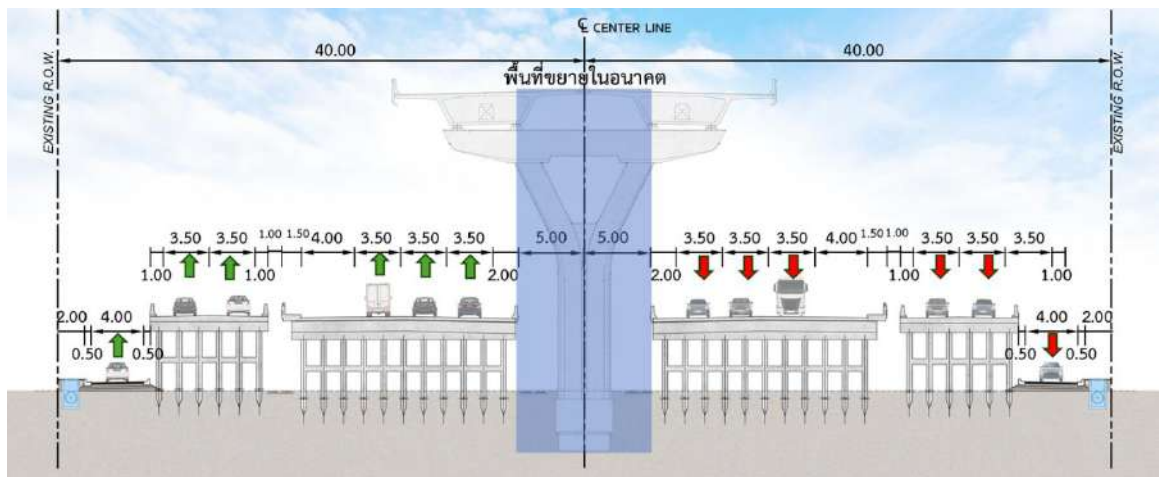
รูปที่ 5-4 ตัวอย่างรูปแบบทั่วไปของถนนโครงการช่วงบริเวณสะพานพร้อมจุดกลับ
