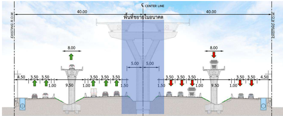
รูปที่ 5-5 ตัวอย่างรูปแบบทั่วไปของถนนโครงการช่วงบริเวณสะพานกลับรถเกือกม้า
