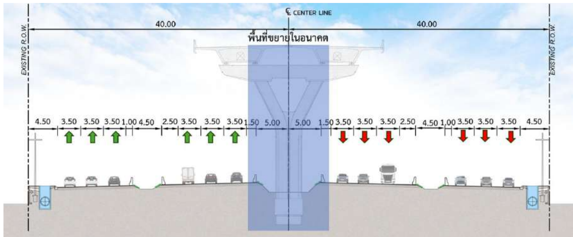
รูปที่ 5-2 ตัวอย่างรูปแบบทั่วไปของถนนโครงการ
