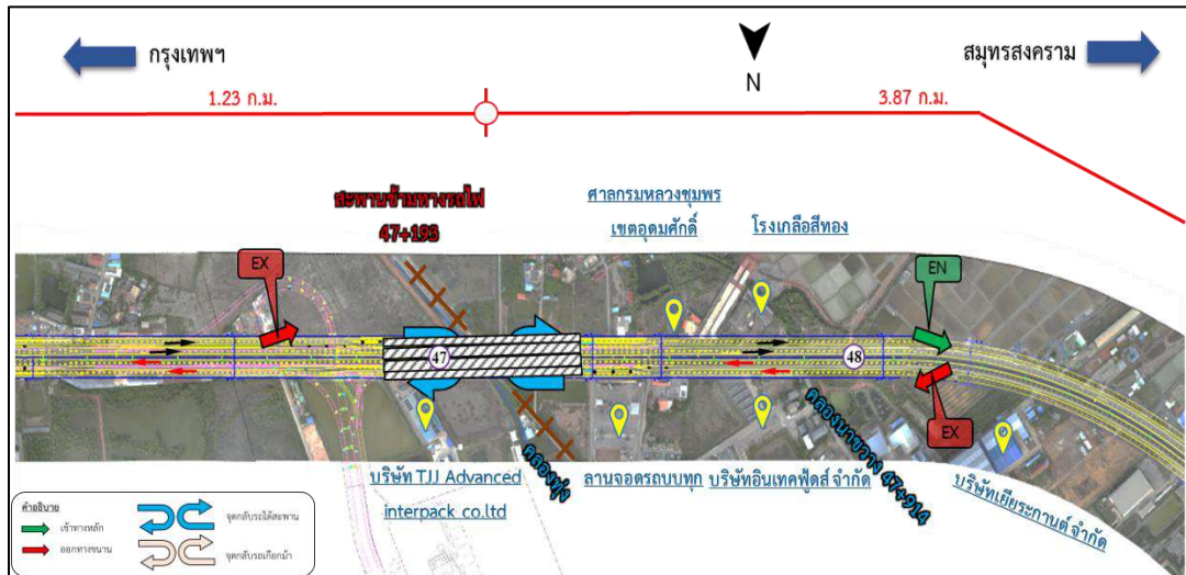
ช่วง บริเวณทางโค้ง กม.49 ถึง จุดกลับรถระดับดิน กม.51+000 (หน้า TRF)
