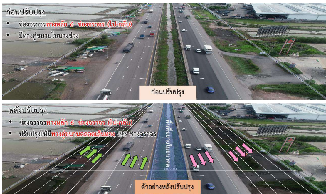
รูปที่ 5-1 รูปแบบตัวอย่างหลังการปรับปรุงเบื้องต้น
