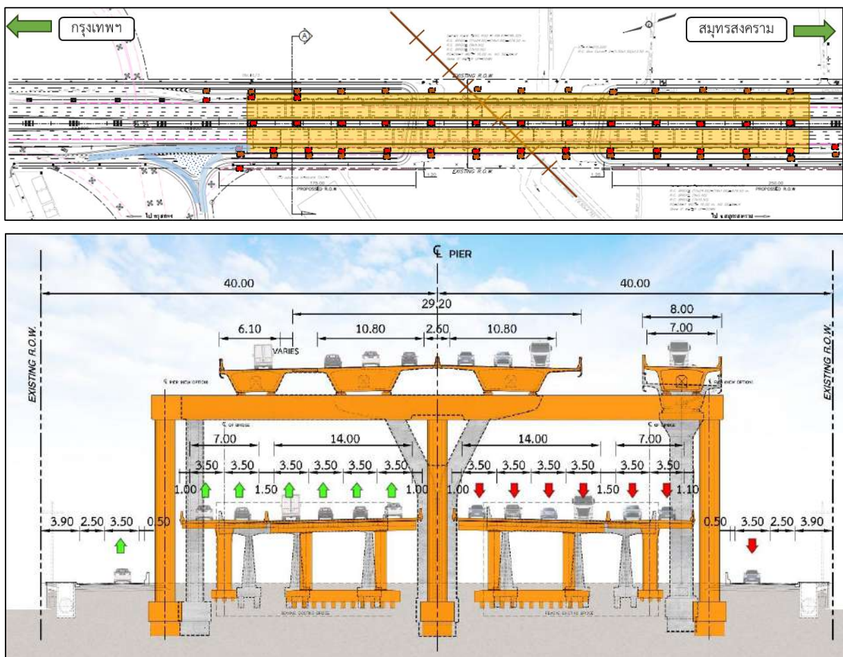
รูปที่ 5-14 รูปแบบทางแยกต่างระดับที่เหมาะสมบริเวณสะพานข้ามทางรถไฟ
